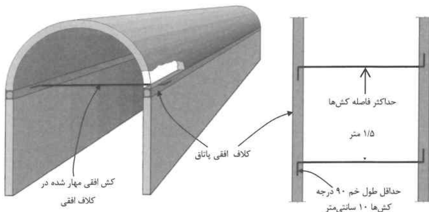
شکل ۷-۳۱ تعبیه مهاربندهای افقی در پاتاق‌های قوسی استوانه‌ای
