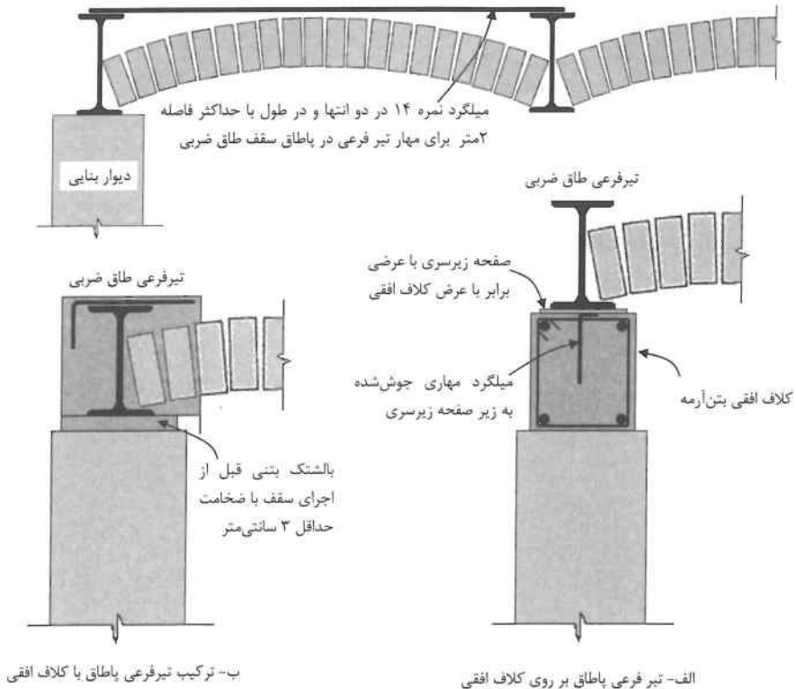
الف- تیر فرعی باطاق بر روی کلاف افقی
