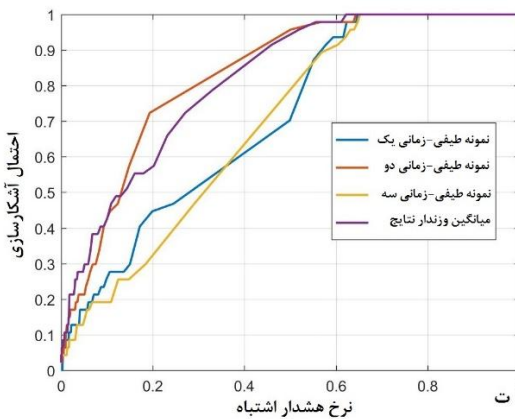
شکل ۱۱: نمودار ROC مربوط به بهینه سازی برای سه طیف انتخابی و میانگین نتایج برای روش های آشکارسازی معرفی شده: الف) CEM (ب) ACE (پ) MF (ت) ASMF
