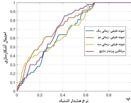
شکل ۱۱: نمودار ROC مربوط به بهینه سازی برای سه طیف انتخابی و میانگین نتایج برای روش های آشکارسازی معرفی شده: الف) CEM (ب) ACE (پ) MF (ت) ASMF
